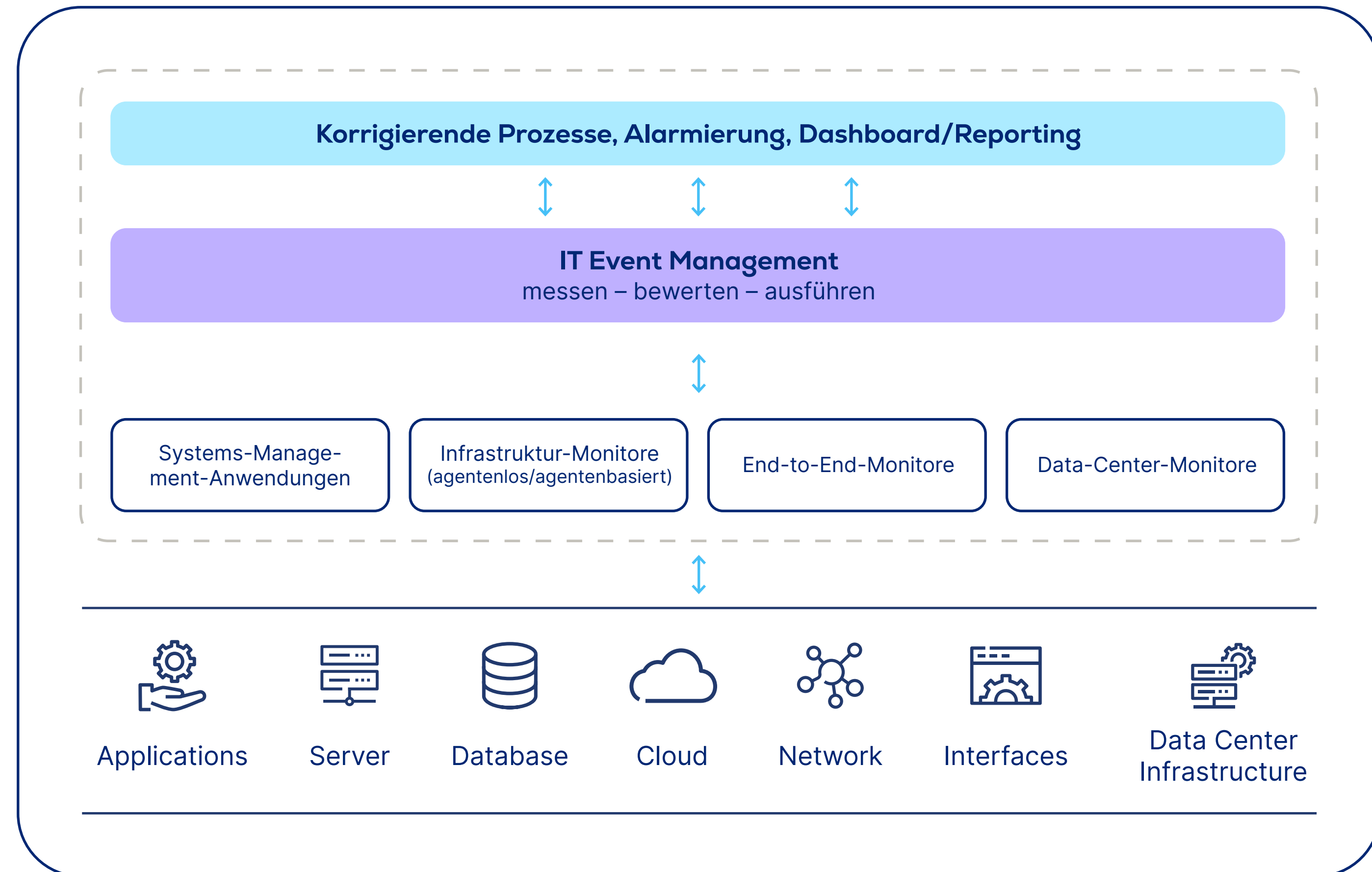
Abbildung 1: Event Management der USU als Herzstück des Monitorings
