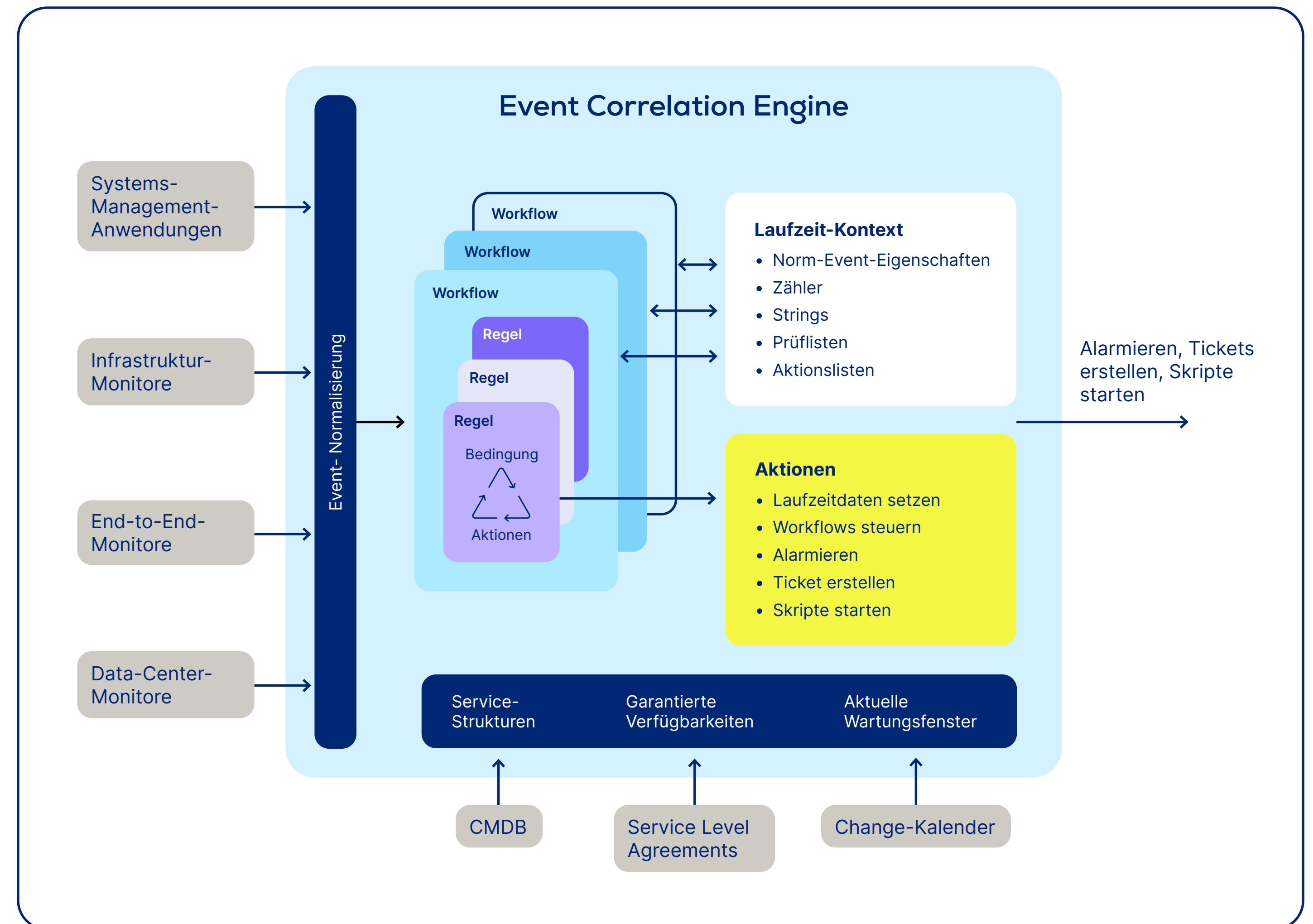
Abbildung 6: Regelbasierte Event-Korrelation der USU
