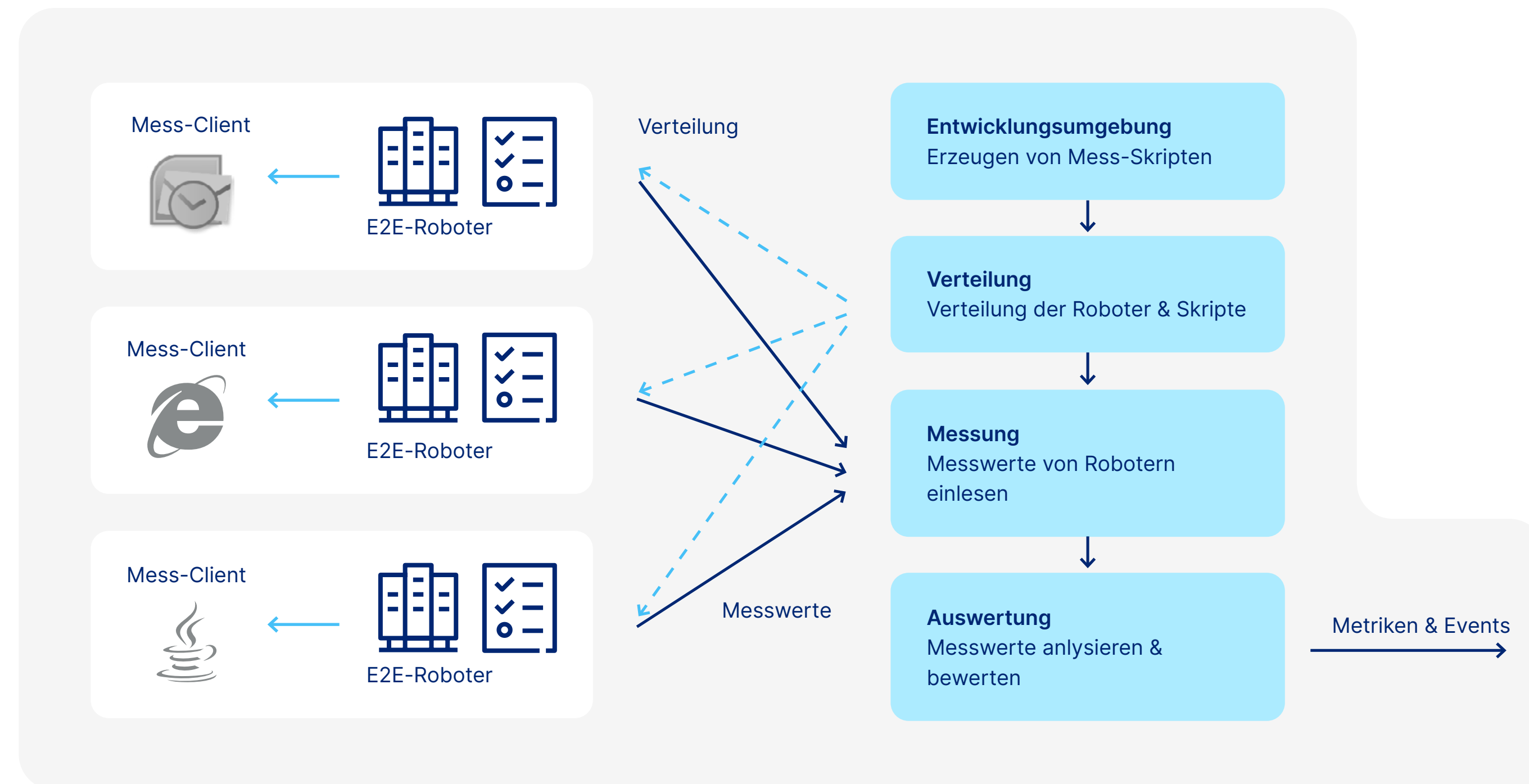
Abbildung 3: End-to-End Monitoring der USU
