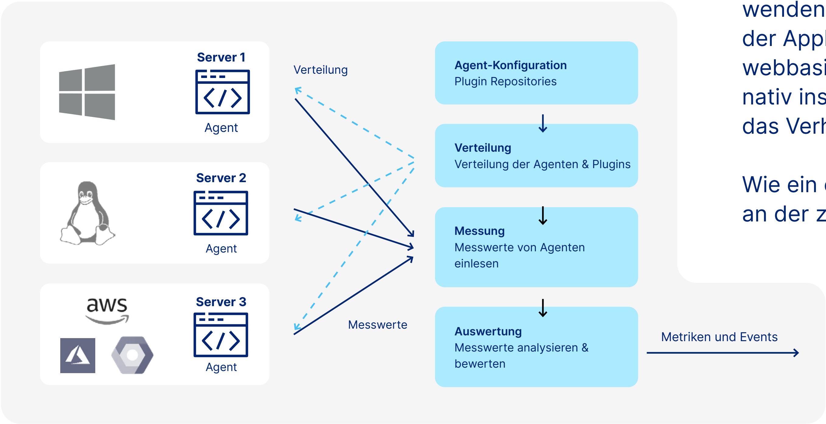
Abbildung 2: Agenten-basiertes Monitoring der USU
